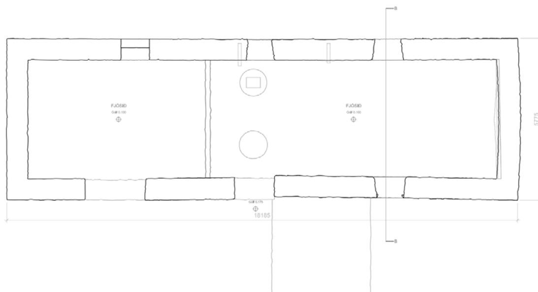
Grunnteikning af fjósinu frá Gullinsniði:
