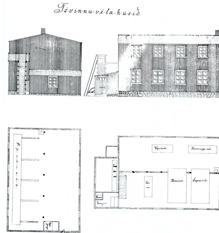
Teikning af tóvinnuhúsinu í Ólafsdal frá árinu 1906 eftir Þorstein Tómasson.
