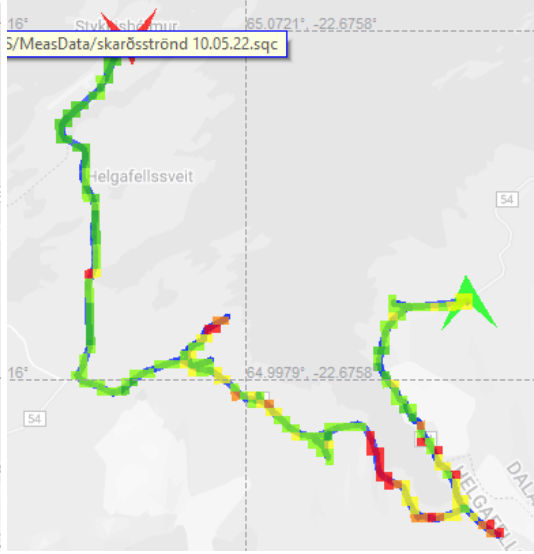
LTE Vodafone/Nova
