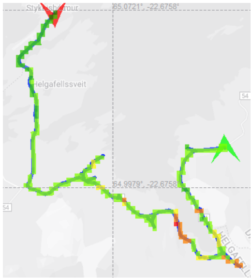
GSM síminn
