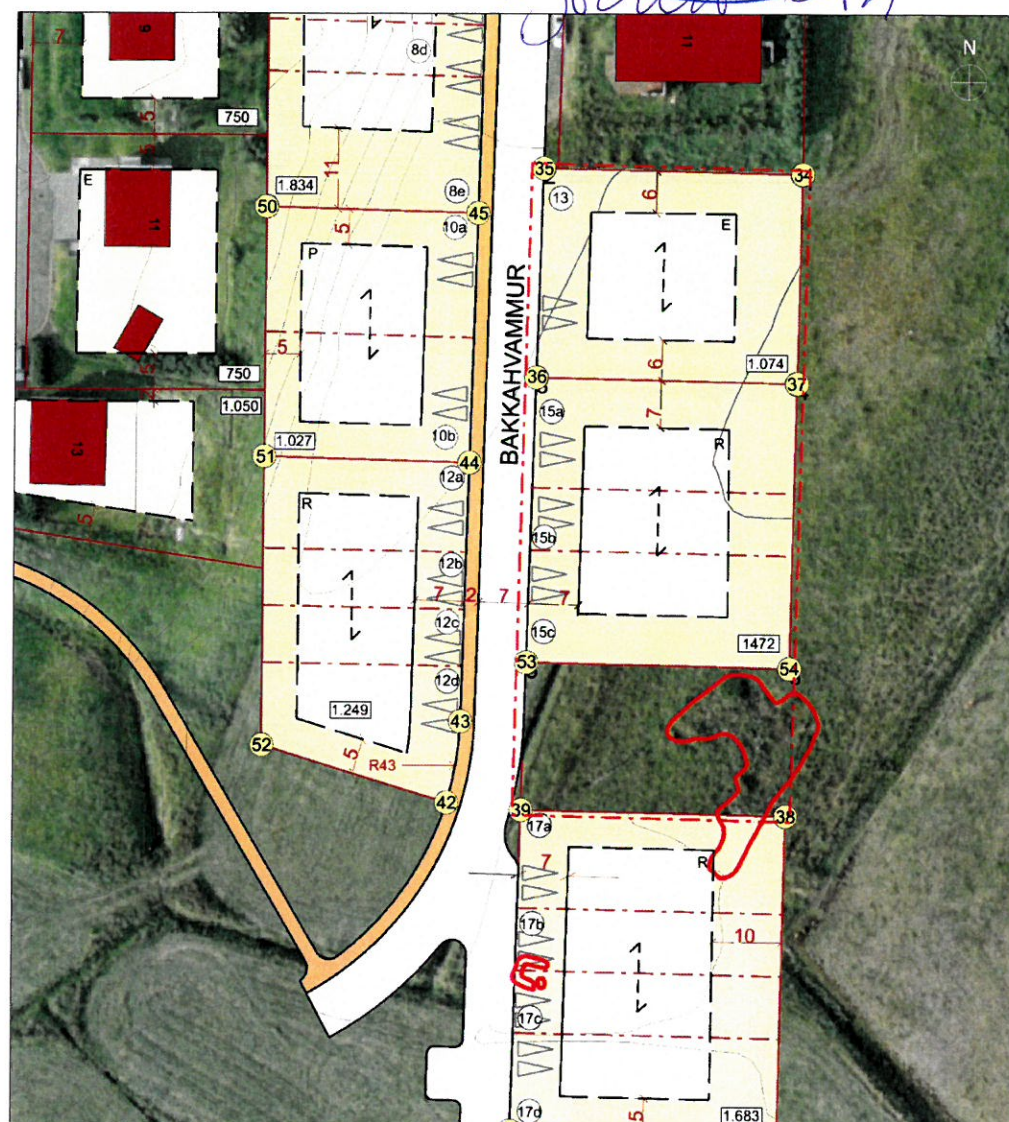
Breyttur deiliskipulagsuppráttur 1:1000
