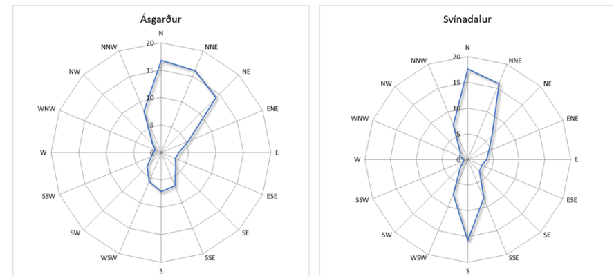
Mynd 3-4 Tíðni vindátta í Ásgarði og Svínadal, meðaltal árunna 2010-2019. 6
