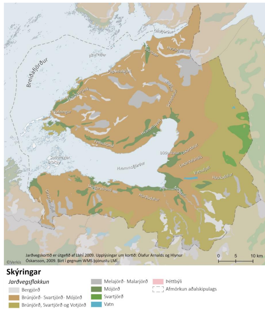
Mynd 3-6 Jarðvegskort af Dalabyggð.
